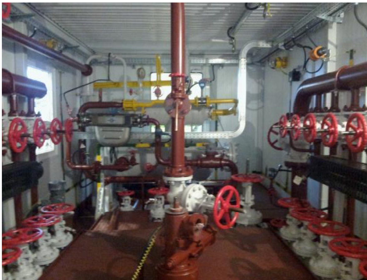
Рисунок 1 - Установка измерительная «Мера-ММ.81». Общий вид
